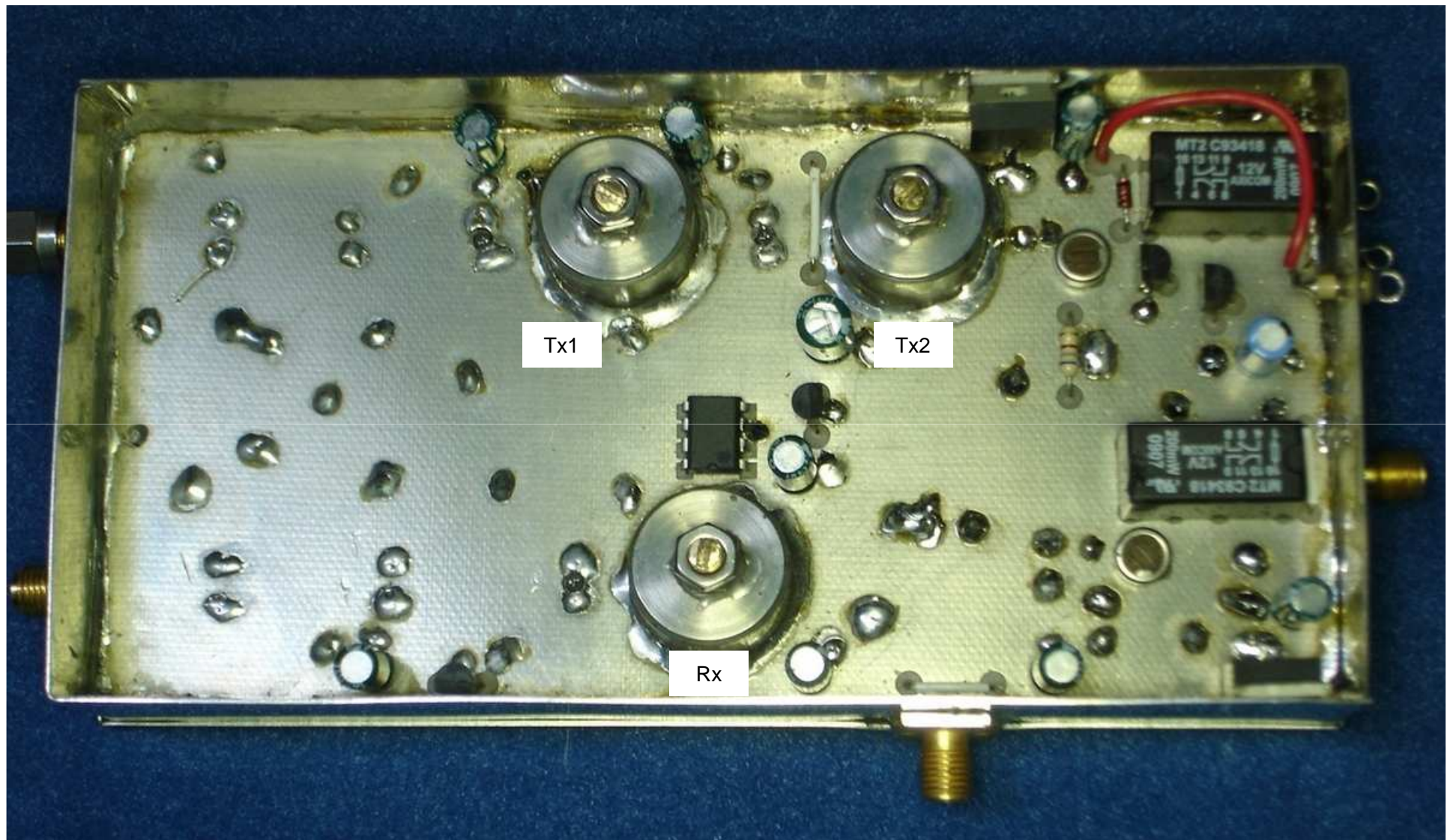
Transverter 10 GHz F1JGP (vers. 1)
