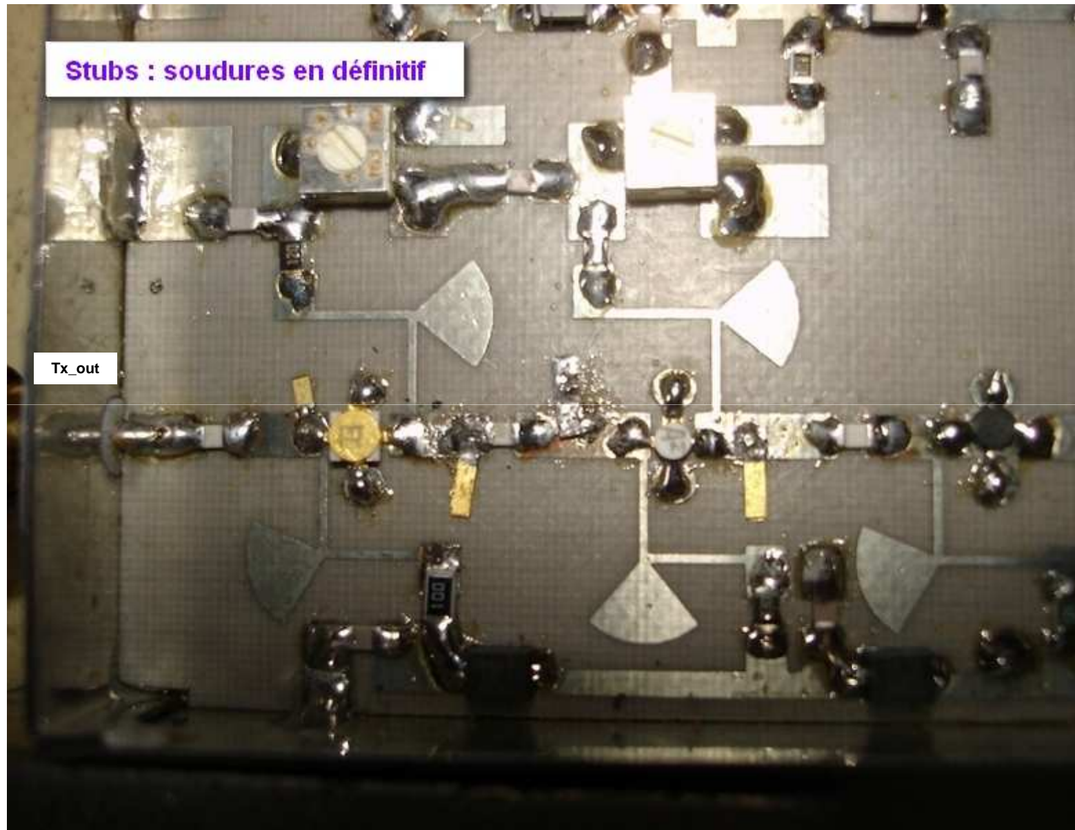
Transverter 10 GHz F1JGP (vers. 1)
