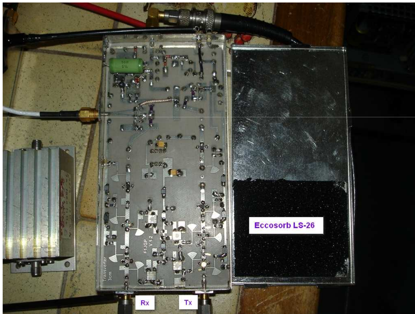
Transverter 10 GHz F1JGP (vers. 1)
