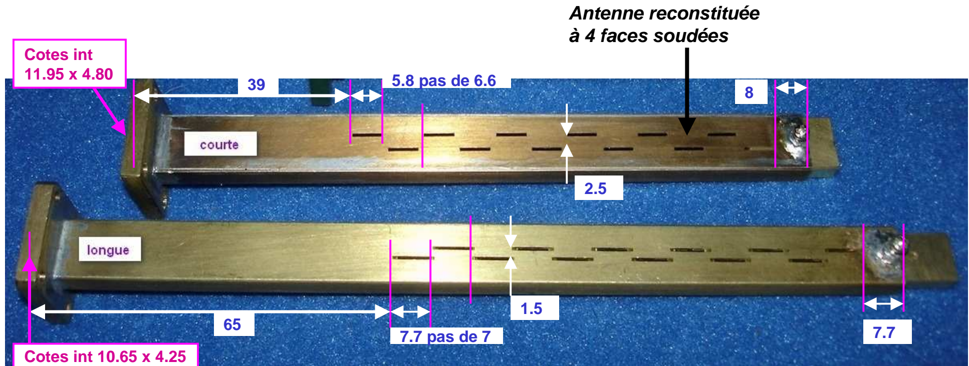
Antenne en vrai WR42
